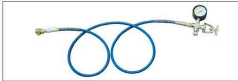
●高圧充填ホース2mヨークゲージ付 No. C505 0000201 ●ホースの長さ2m
